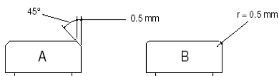
Figure 10. Épée: design of pointes d'arrêt
